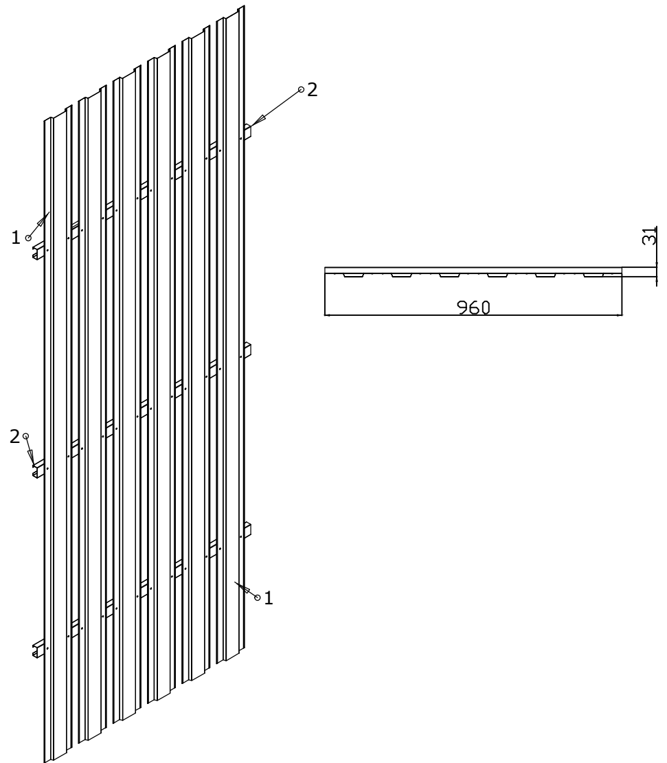
ELEMENTY 1-2 KLINCZOWANE
