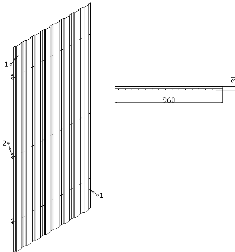
ELEMENTY 1-2 KLINCZOWANE
